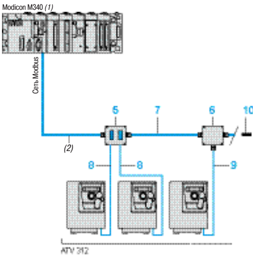
Пример архитектуры сети Modbus, подключение через ответвительную коробку
