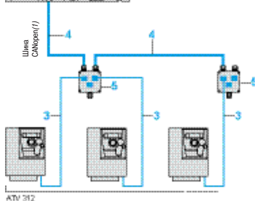
Классическое решение для подключения к шине CANopen установки
