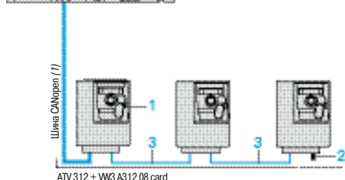
Оптимальное решение для последовательного подключения к шине CANopen установки
