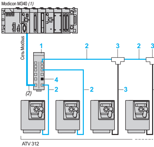
Пример архитектуры сети Modbus, подключение через разветвительный блок и разъемы RJ45
