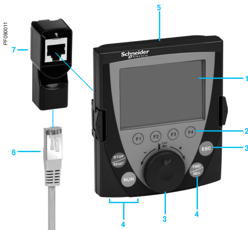
Выносной графический терминал + адаптер RJ45 + Удлинительный кабель
