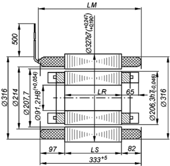
Габаритные, установочные и присоединительные размеры двигателя АИРРВВ200В4УХЛ2. Монтажное исполнение IM 5010
