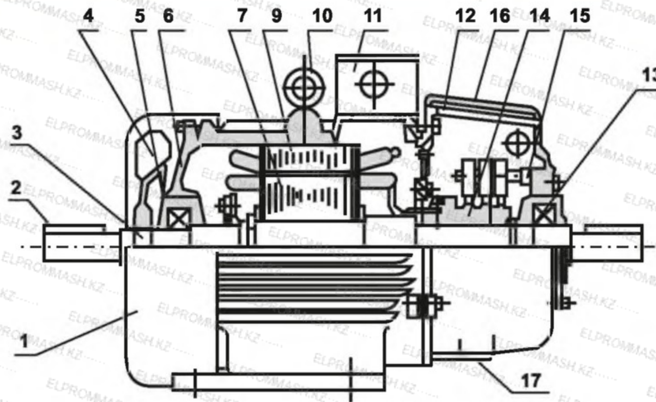
Рис. 2 Конструкция электродвигателя с фазным ротором
