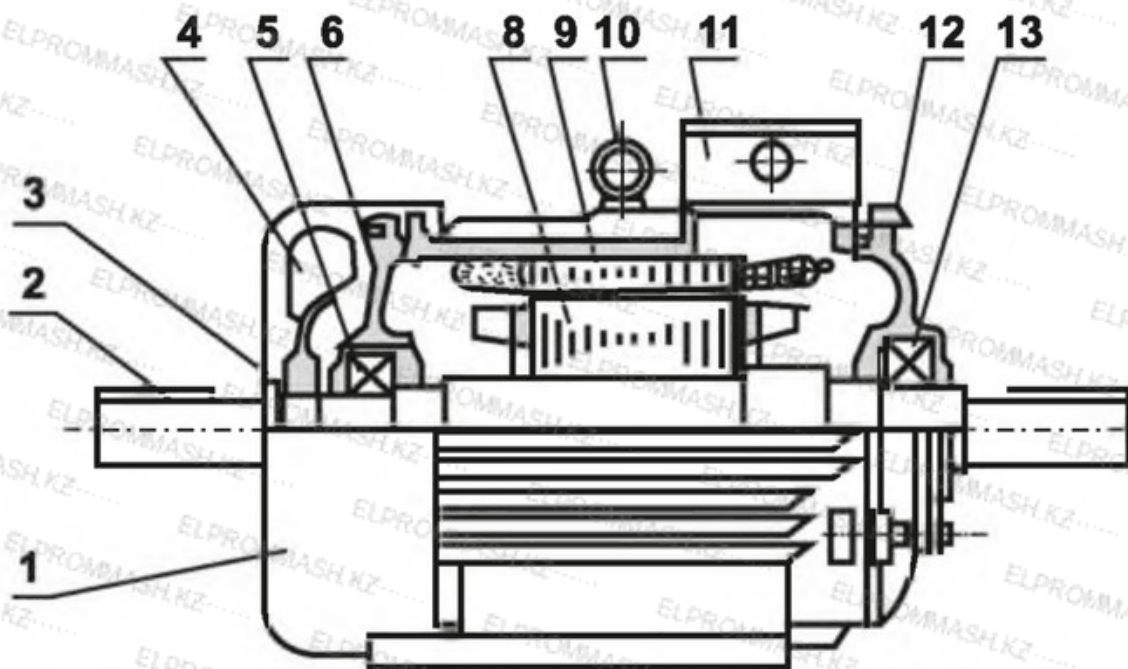
Рис. 3 Конструкция электродвигателя с короткозамкнутым ротором
