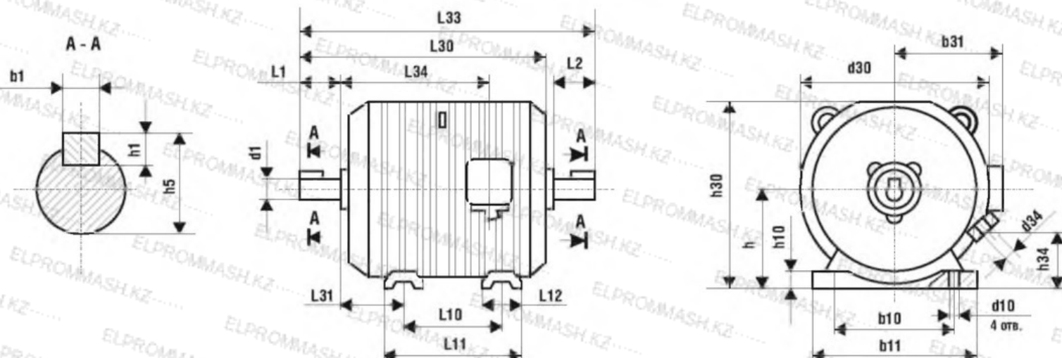
Конструктивное исполнение IM1001
