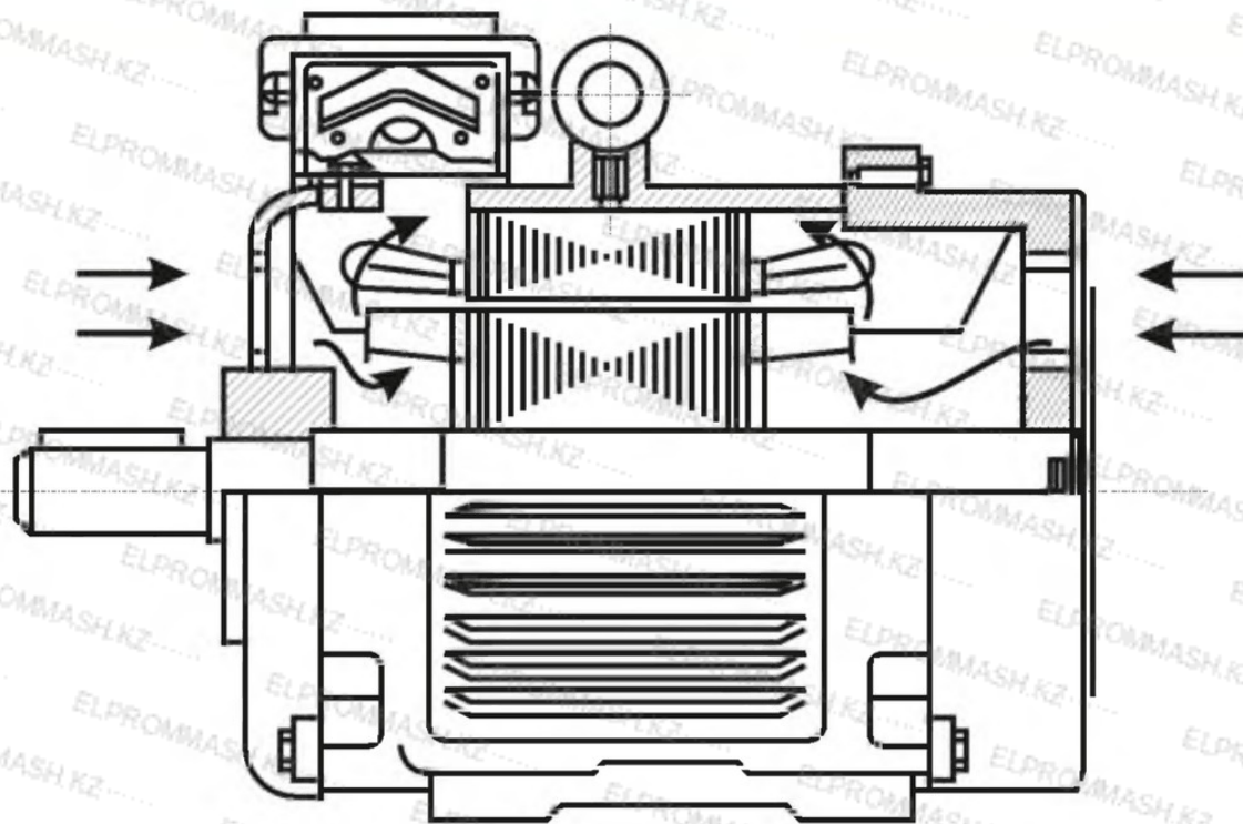
Рис. 1 Конструкция электродвигателя брызгозащищенного исполнения
