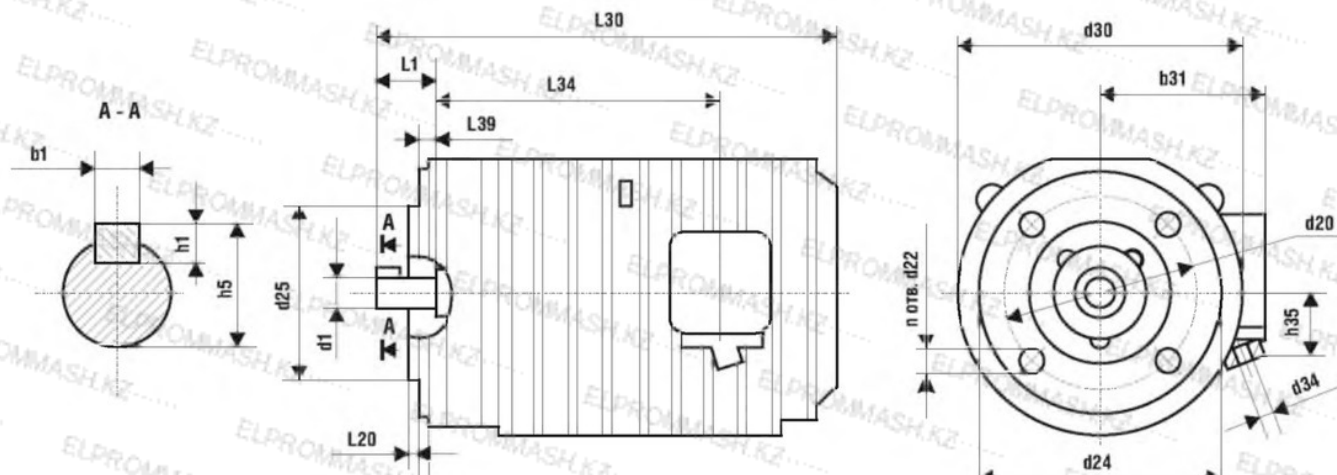
Конструктивное исполнение IM3001
