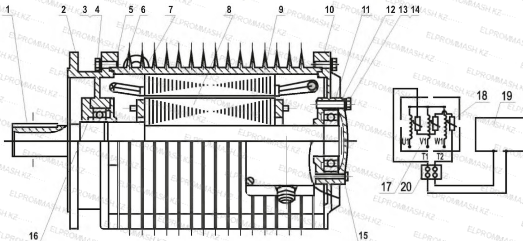
Рис. 5 Конструкция рольганговых электродвигателей
